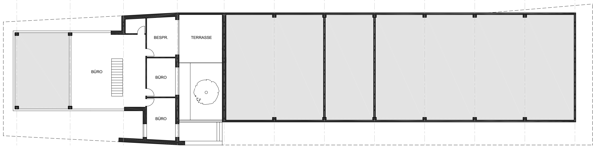
obergeschoss
